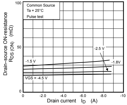
R_{DS(ON)} - I_D
