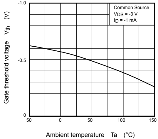
V_{th} - T_a
