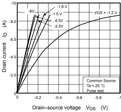
I_D - V_{DS}
